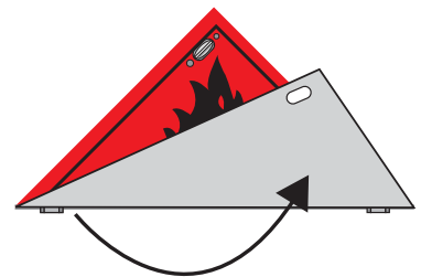
Panneau pour symboles ADR, à articulation horizontale
